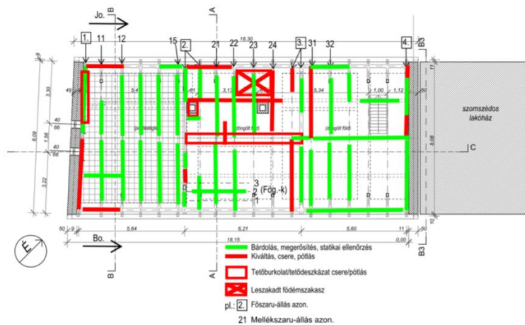
Részletes kárjegyzék alapján készített pontos kártérkép a tetőszerkezet károsodott elemeiről
